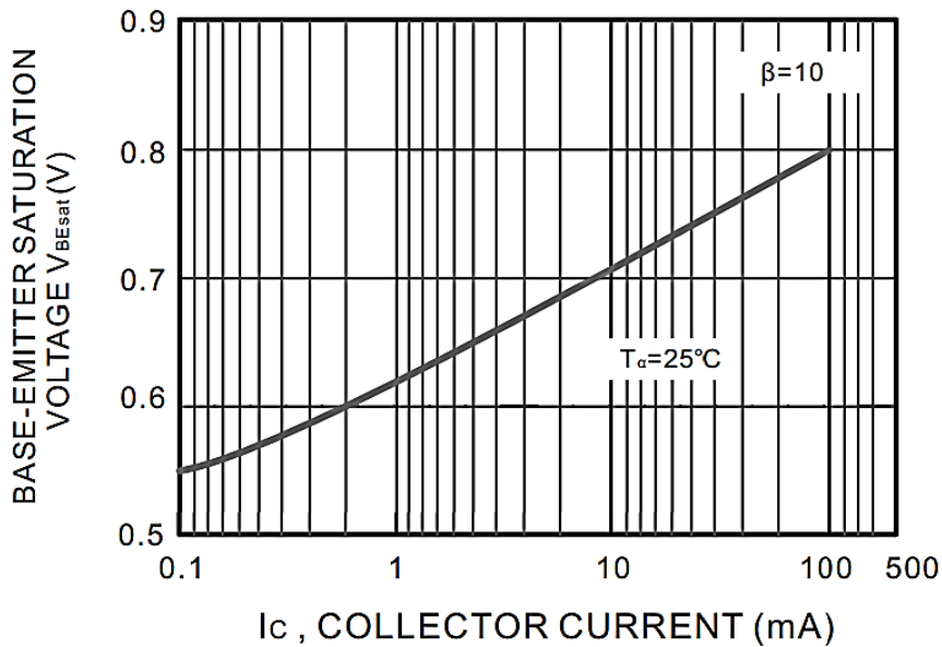
Fig.6 V_{BEsat} - I_c
