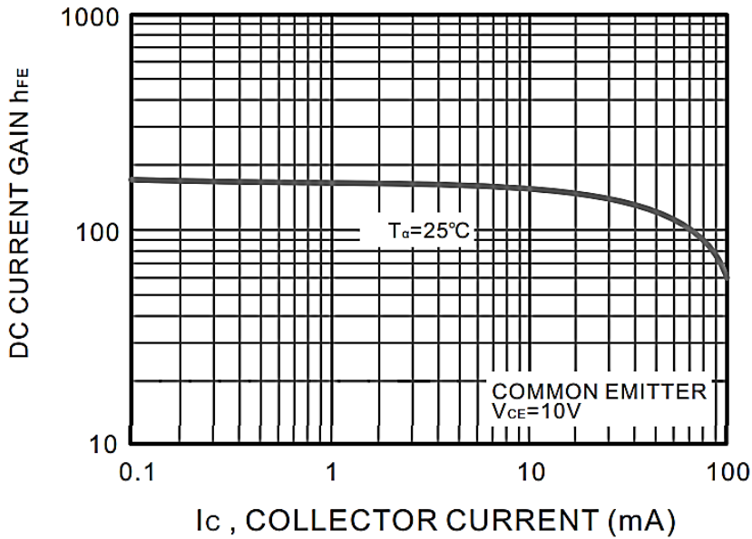
Fig.5 h_{FE} - I_c
