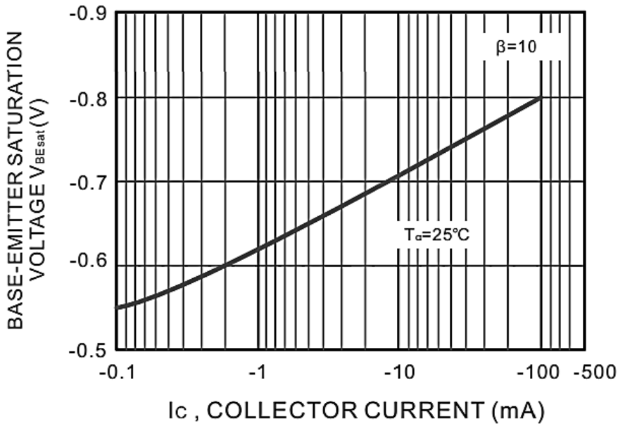
Fig.6 V_{BEsat} - I_c
