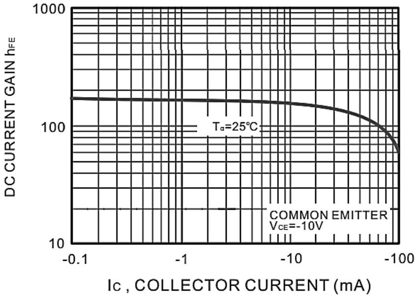
Fig.5 h_{FE} - I_c
