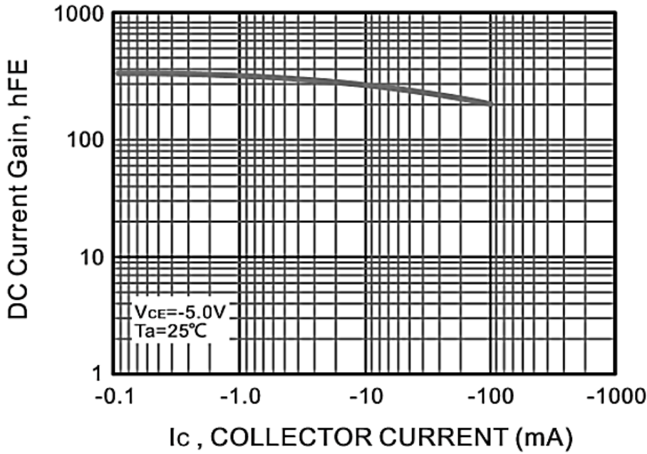
Fig.3 h_{FE} -- I_c
