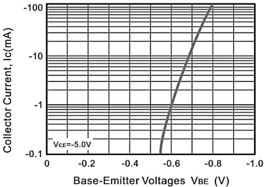
Fig.4 I_c -- V_{BE}
