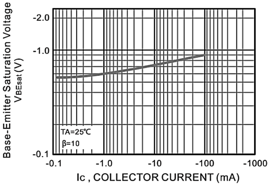
Fig.5 V_{BEsat}--I_c
