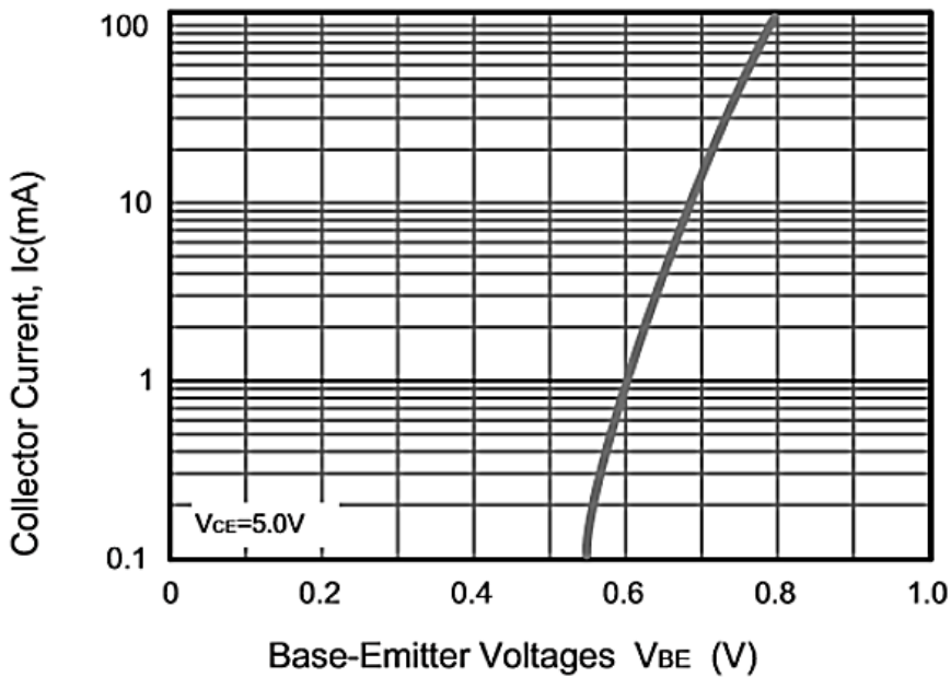
Fig.4 I_c-V_{BE}
