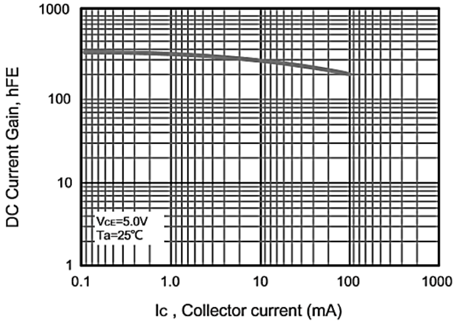
Fig.3 h_{FE}-I_c
