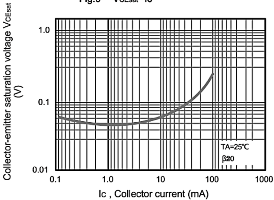
Fig.6 V_{CEsat}-I_c
