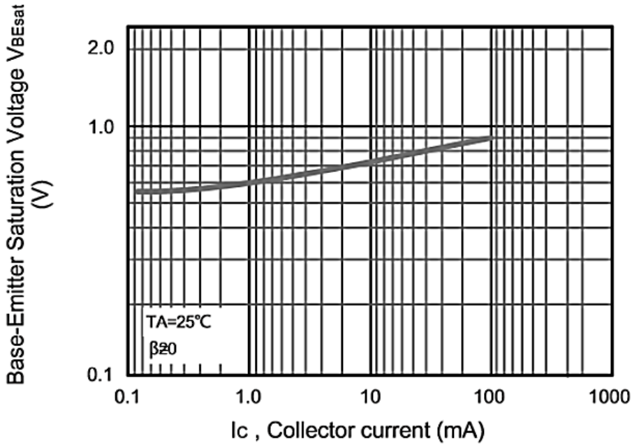
Fig.5 V_{BEsat}-I_c
