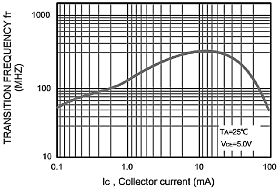
Fig.7 f_T - I_C
