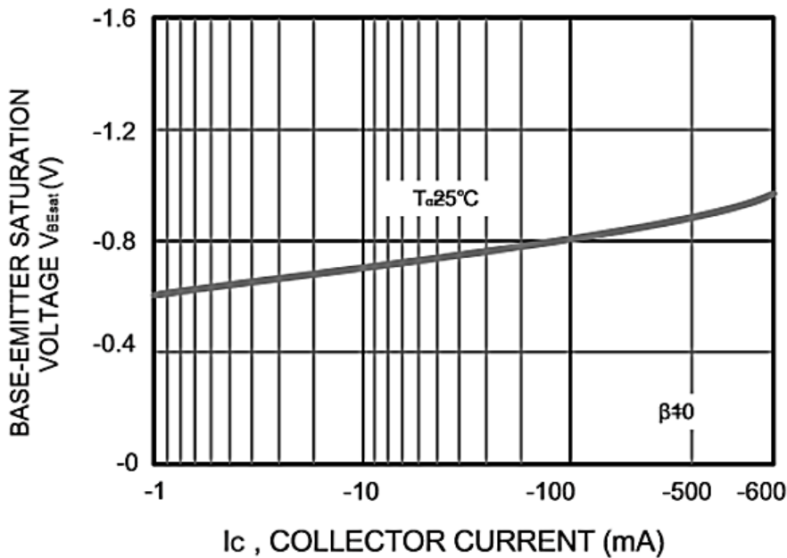
Fig.6 V_{BEsat} - I_c
