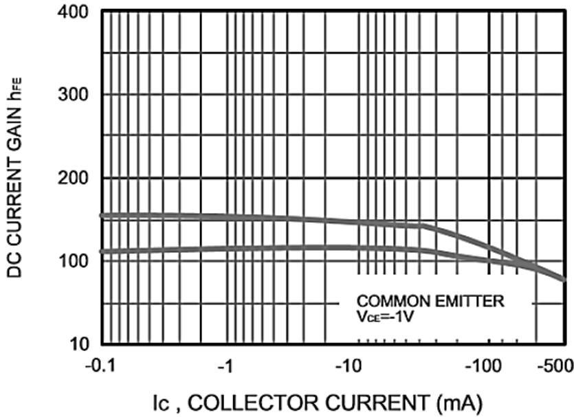
Fig.5 h_{FE} - I_c
