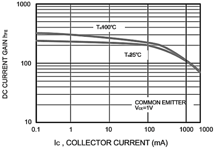
Fig.5 h_{FE}-I_c
