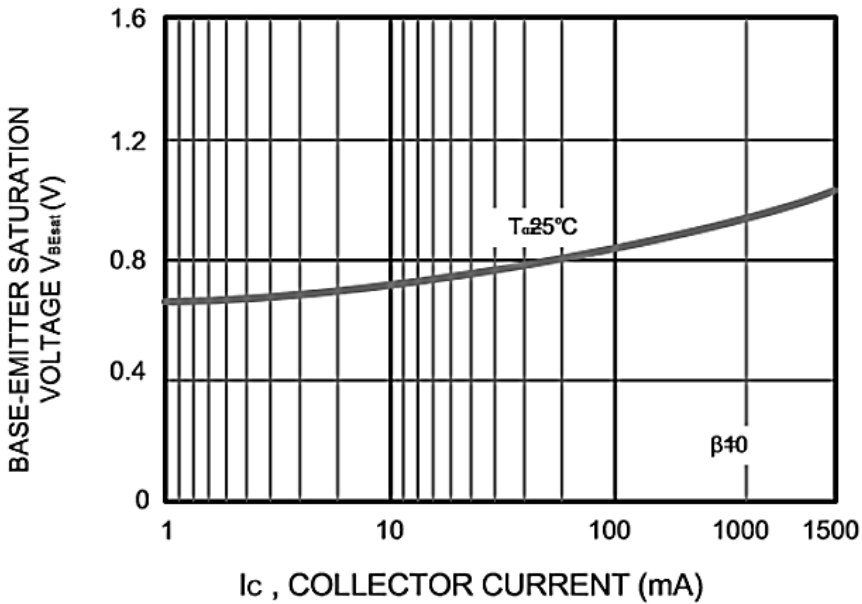
Fig.6 V_{BEsat}-I_c
