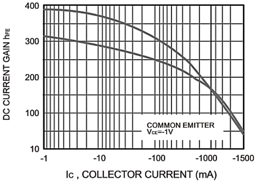
Fig.5 h_{FE}-I_c
