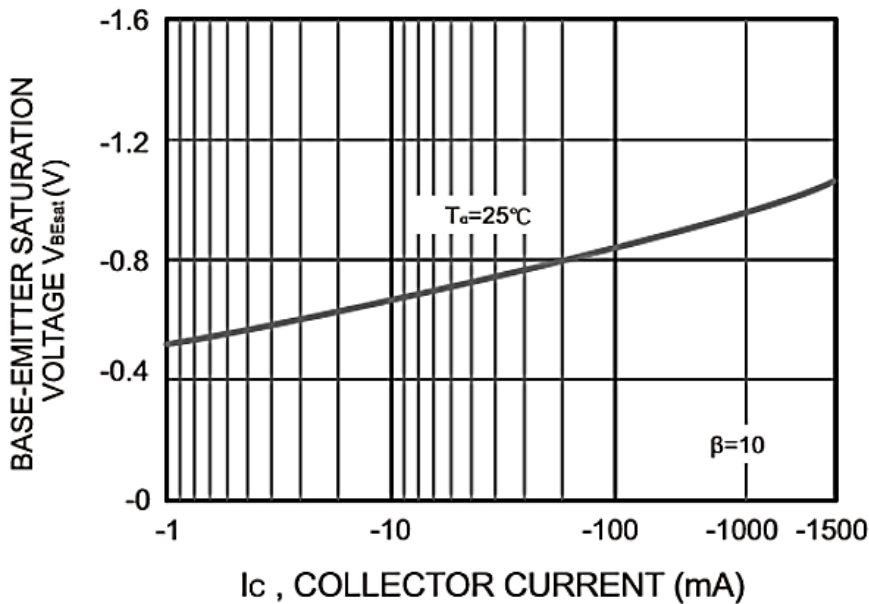
Fig.6 V_{BEsat}-I_c
