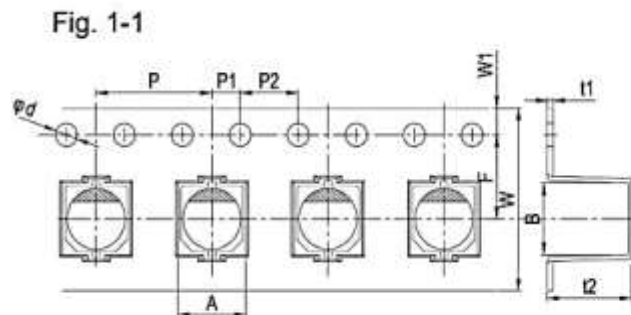
Fig. 1 ( \varnothing 4 \sim \varnothing 10 )
