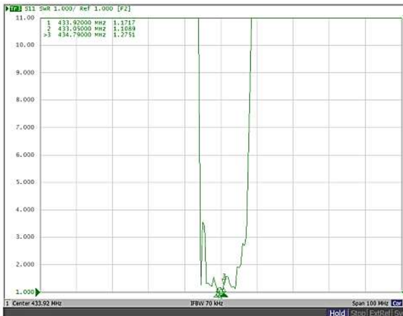
S11 VSWR
