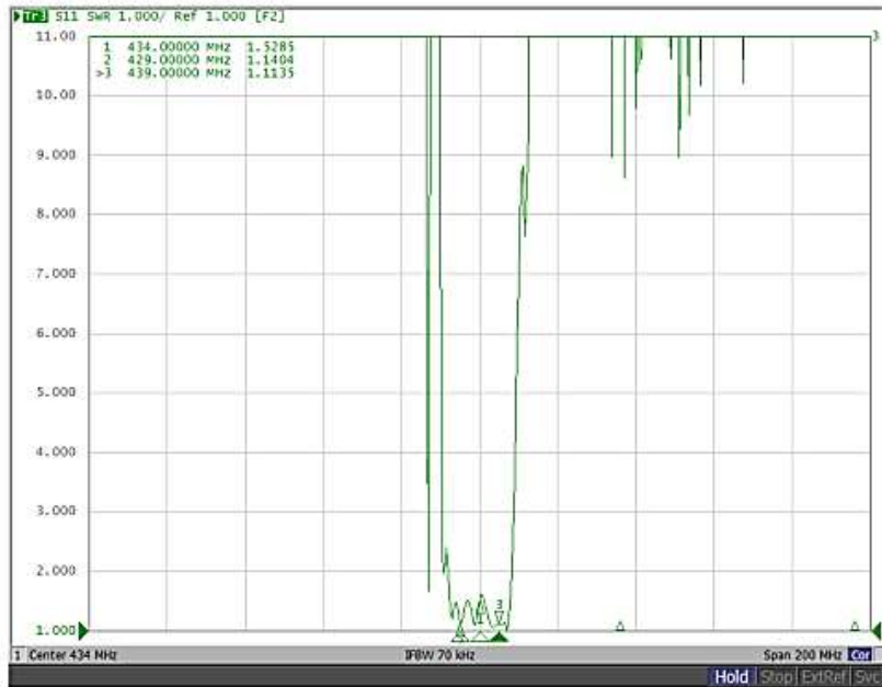
S11 VSWR
